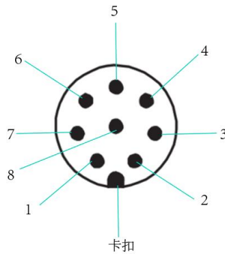
图 3.2 末端 I/O 插座引脚分布
