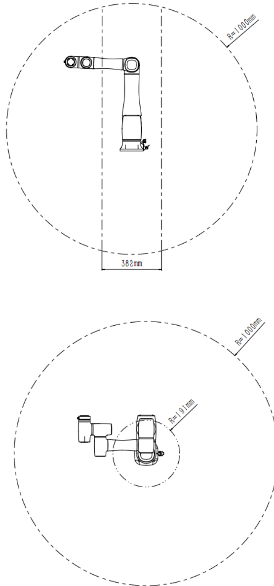
图 2.6 工作范围
