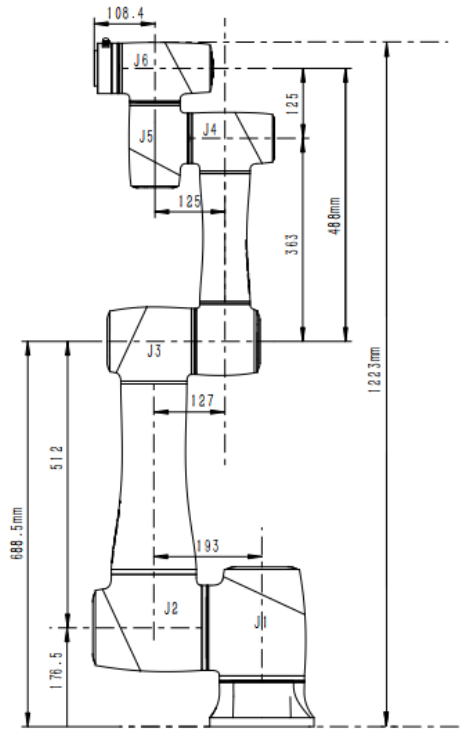
图 2.2 本体尺寸
